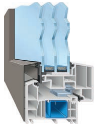
AFINO-art AD (Anschlagdichtungssystem mit zwei Dichtungen)
