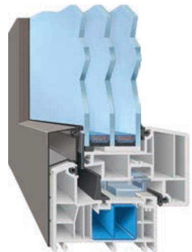
AFINO-art MD (Mitteldichtungssystem mit drei Dichtungen)
