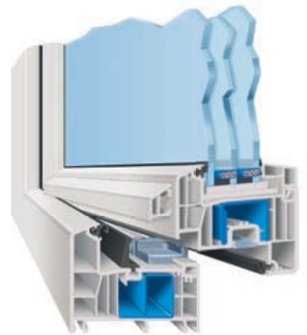
AFINO-one MD (Mitteldichtungssystem mit drei Dichtungen)
